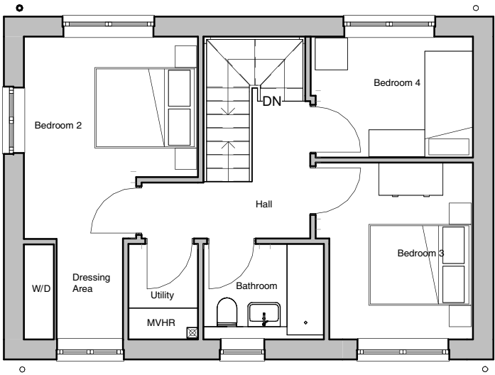
2 Housetype D First Floor 1 : 100
